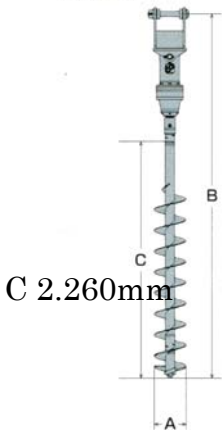
寸法図
